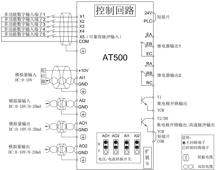
图 3-3 变频器控制回路典型接线示意图
