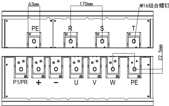
图 3-15 三相 315-450kW 主回路端子分布及尺寸图
