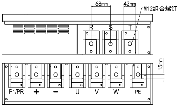
图 3-13 三相 160-200kW 主回路端子分布及尺寸图
