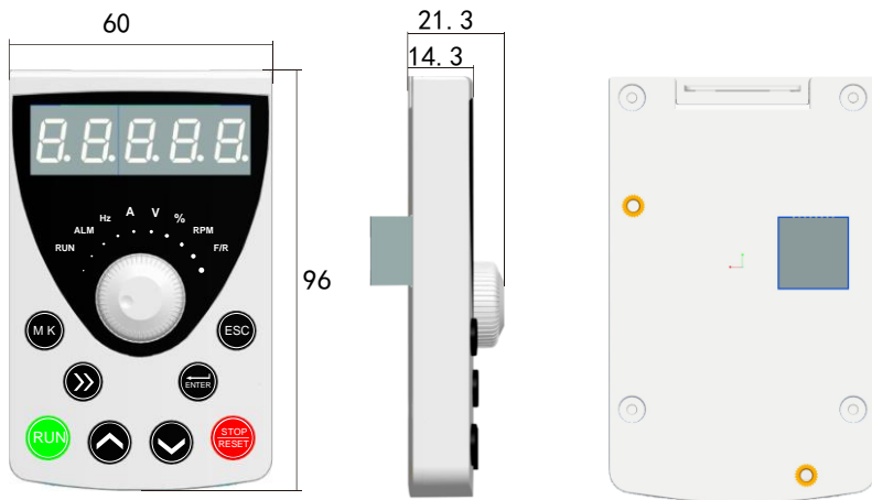
图 1-9 键盘外观及安装尺寸 (mm)
