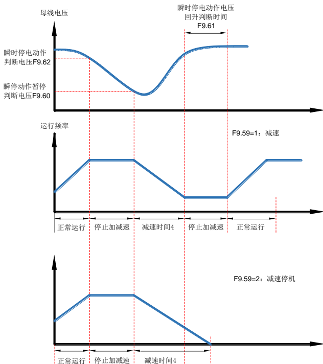
图 7-23 瞬时停电动作示意图
