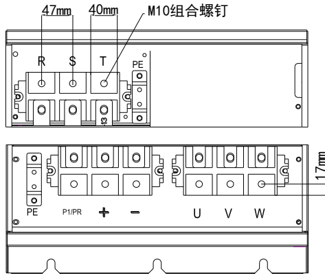
图 3-12 三相 110-132kW 主回路端子分布及尺寸图
