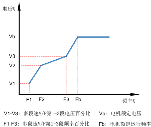
图 7-19 四点 V/f 曲线示意图
