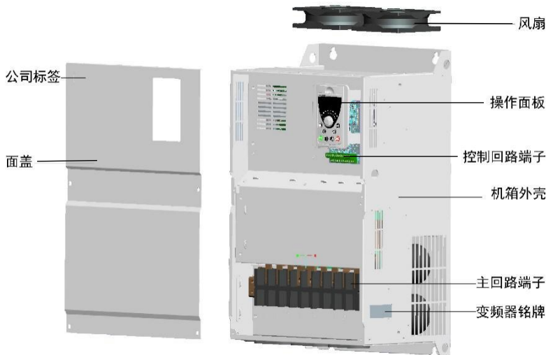
图 1-4 钣金外壳机型各部分名称
