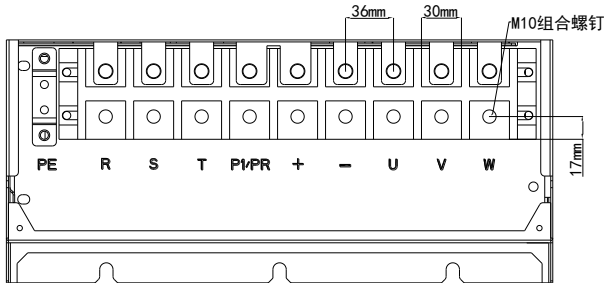
图 3-11 三相 75-90kW 主回路端子分布及尺寸图
