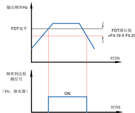
图 7-10 频率 FDT 示意图
