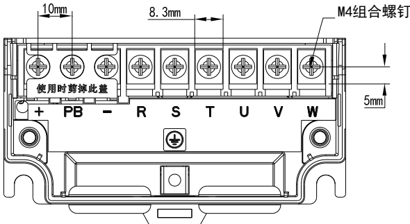
图 3-5 三相 0.75-2.2kW 主回路端子分布及尺寸图
