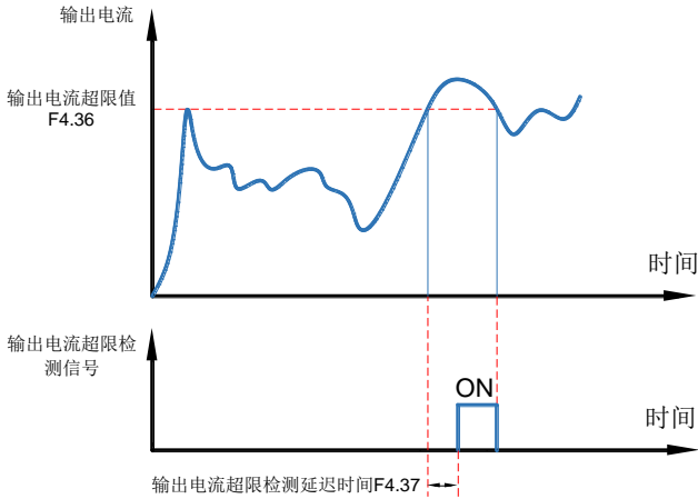
图 7-15 输出电流超限示意图
