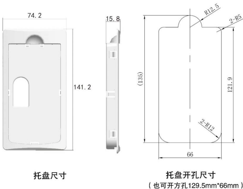
图 1-12 双行键盘托盘外观及开孔尺寸 (mm)
