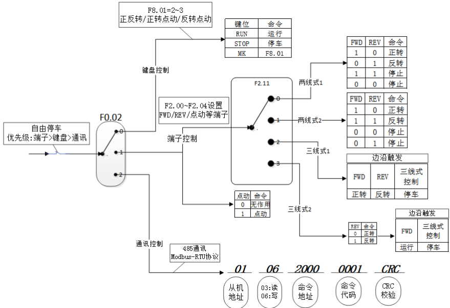
图 5-4 运行命令给定方式选择
