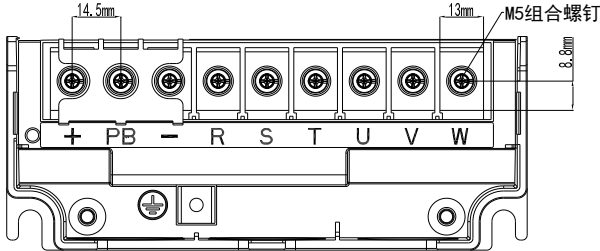
图 3-7 三相 7.5-11kW 主回路端子分布及尺寸图
