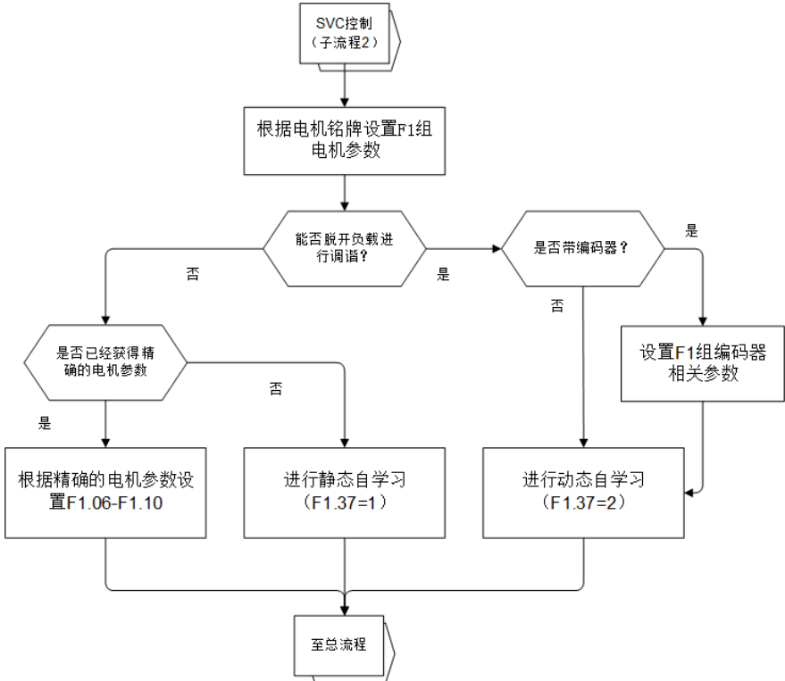
图 5-3 变频器调试试子流程（矢量控制）
