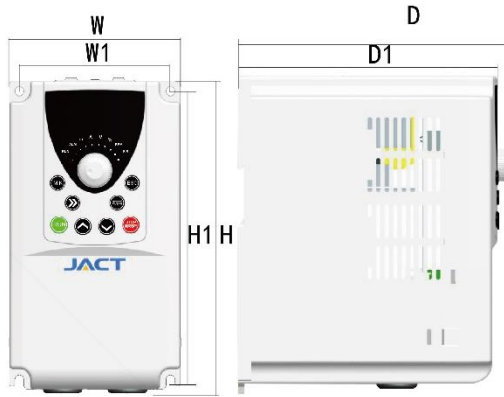
图 1-5 塑壳机器安装尺寸
