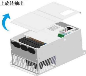
图 2-3 钣金外壳机型盖板拆卸
