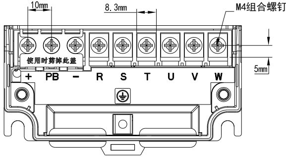
图 3-4 单相 0.75-2.2kW 主回路端子分布及尺寸图
