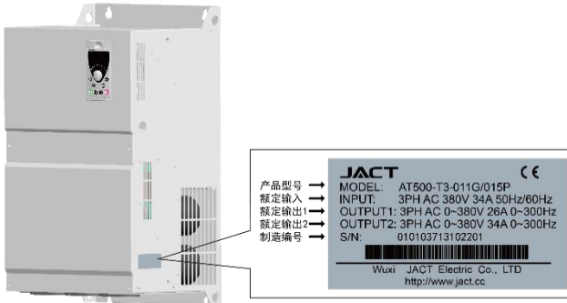
图 1-2 产品铭牌
