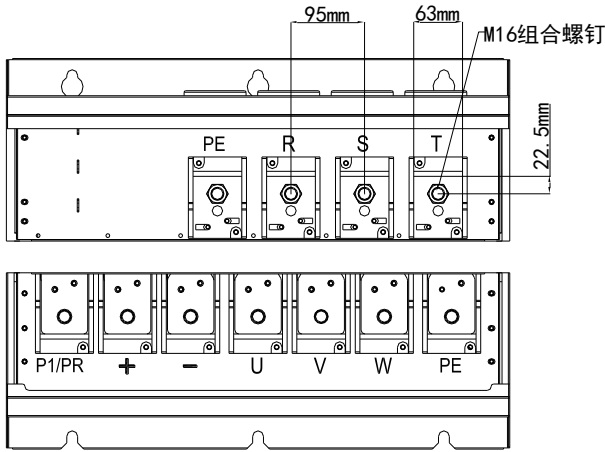
图 3-14 三相 220-280kW 主回路端子分布及尺寸图
