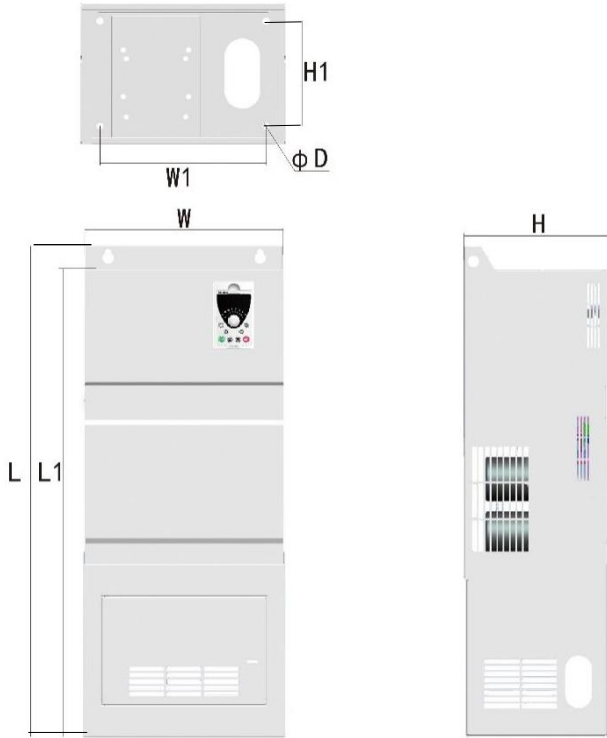
图 1-8 柜式安装尺寸图
