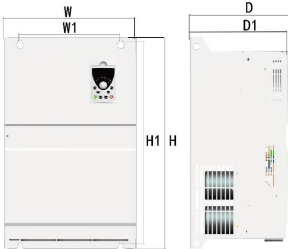
图 1-6 钣金机器安装尺寸
