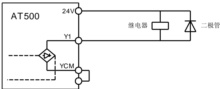
图 3-23 数字输出端子接线示意图
