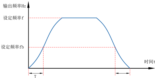
图 7-20 S 加减速曲线 A 示意图
